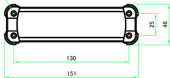
A-A (1:2.5)
